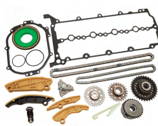
DA3413 Contiene guías, cadenas, tensores, piñones, piñones calado de la distribución y juntas. • Motores Ingenium AJ200D
